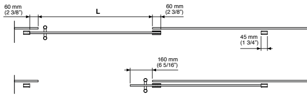
VIDRIO FIJO 10 mm / FIXED GLASS 3/8"
